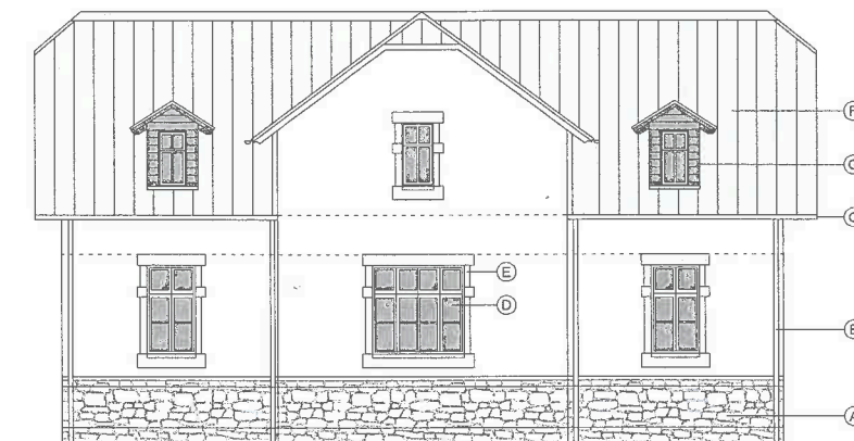
POHLED VÝCHODNÍ
