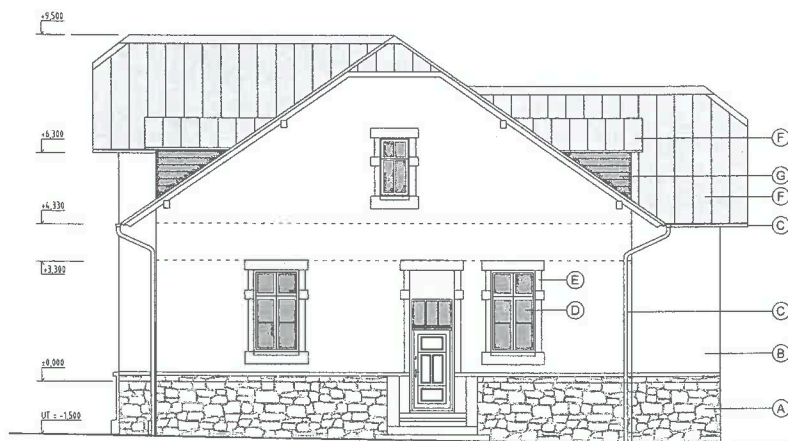
POHLED SEVERNÍ
