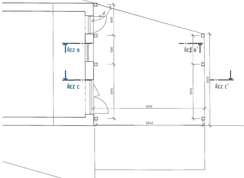
Půdorys 1 NP
