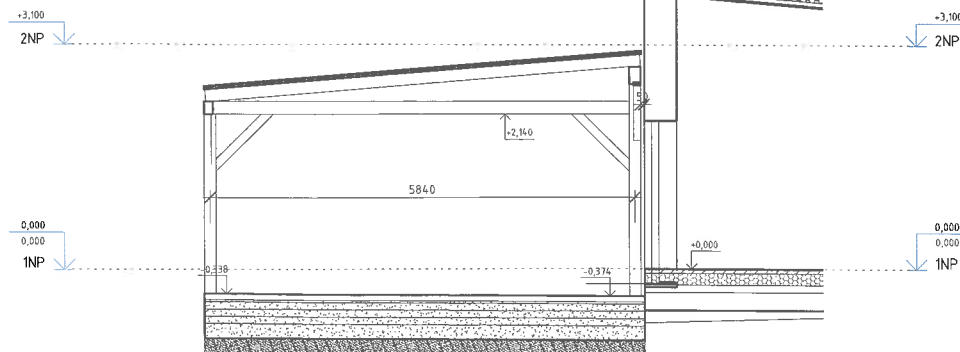
ŘEZ B
