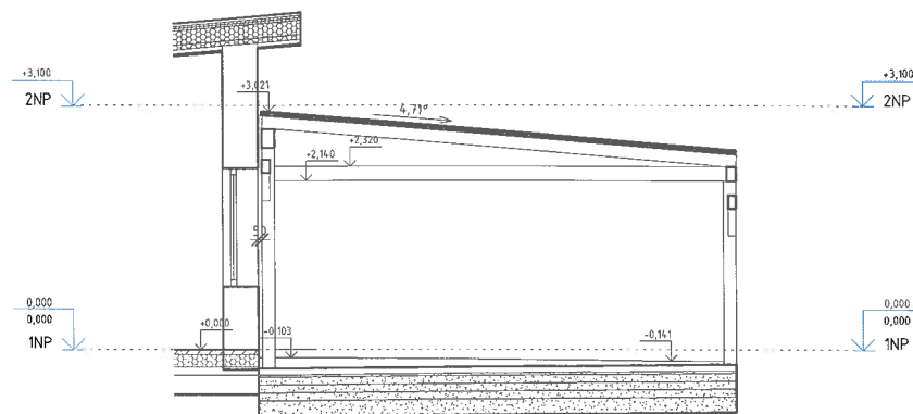
ŘEZ B
